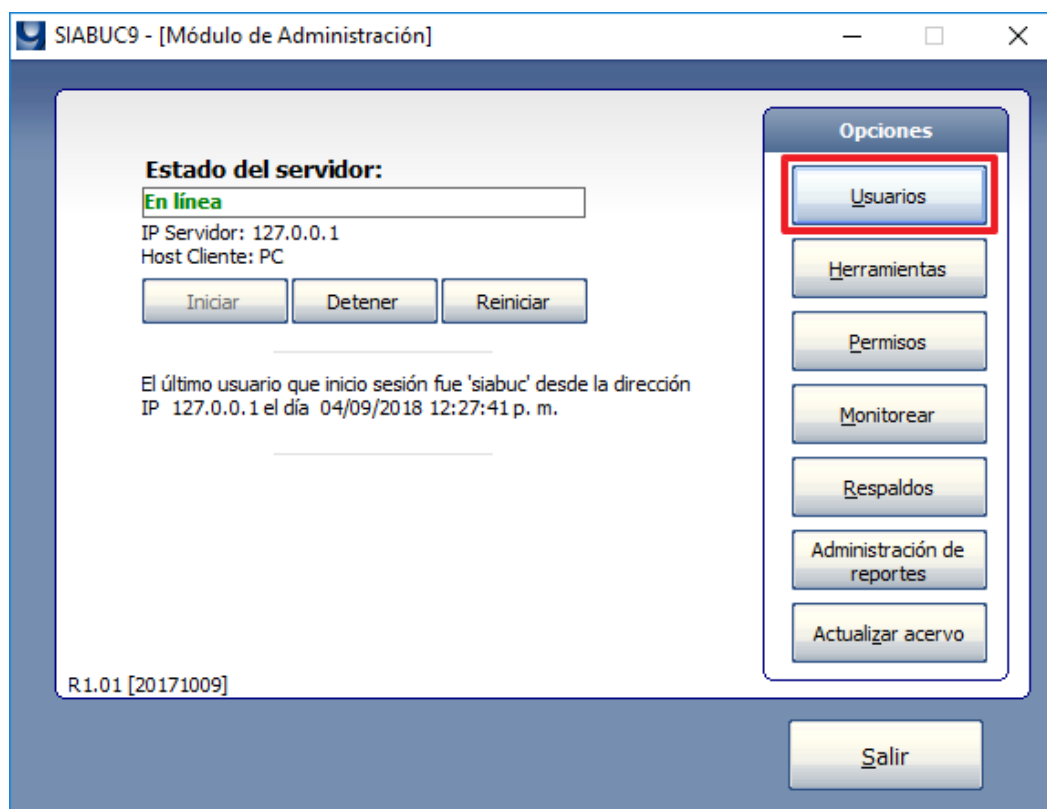
Ilustración 1. Opción Usuarios
