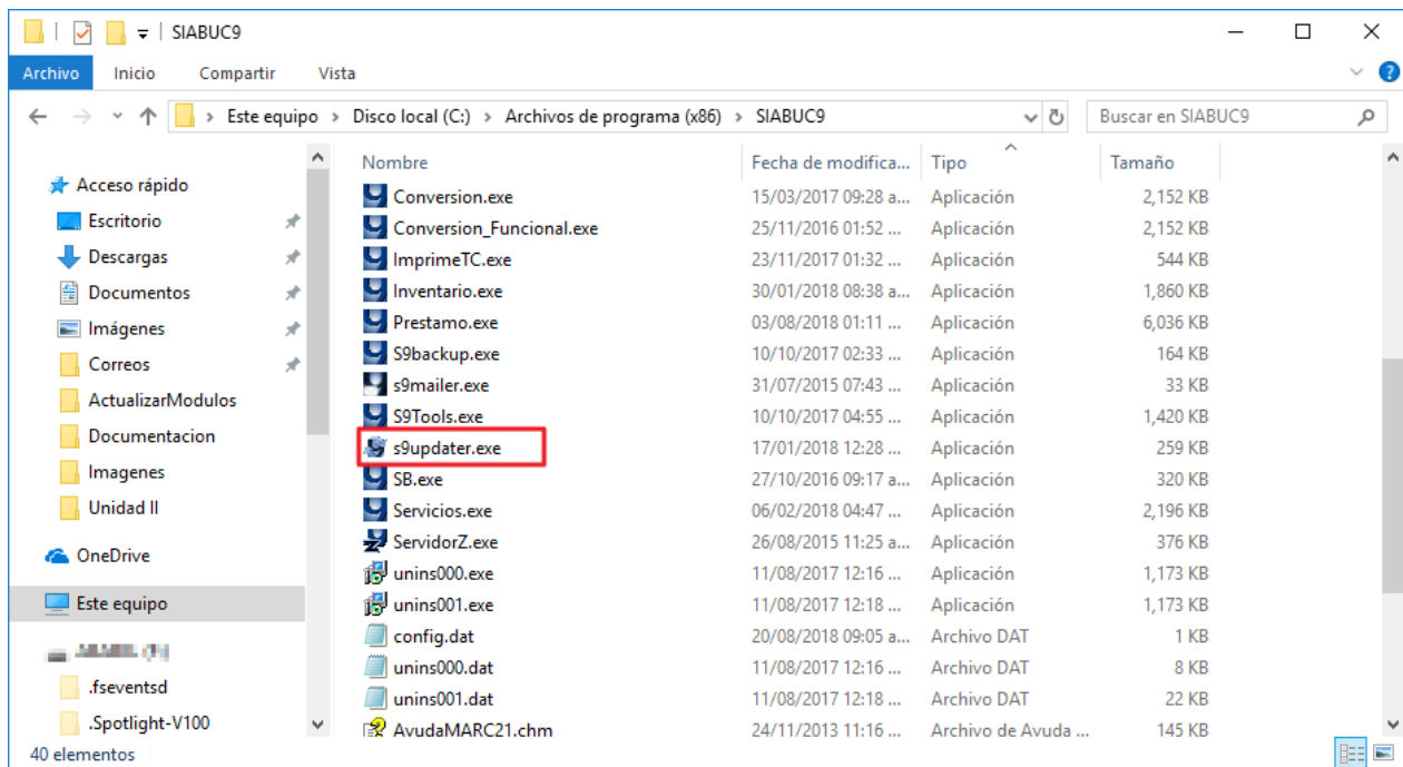
Ilustración 15. Aplicación s9updater.exe
