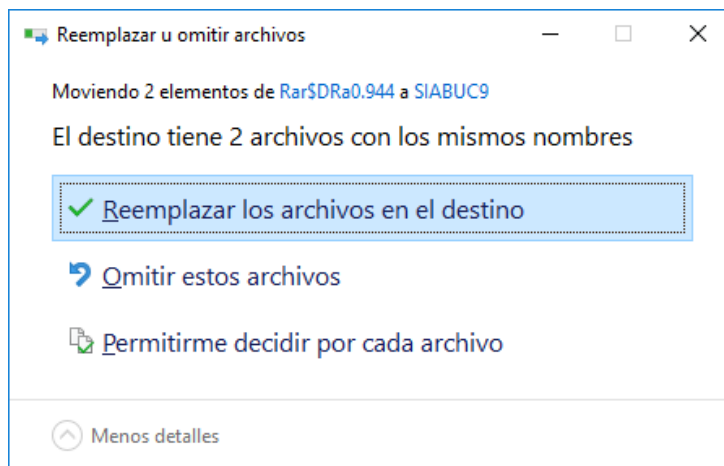
Ilustración 7. Reemplazar archivos
